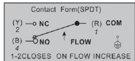
HY68 液位开关接线图
